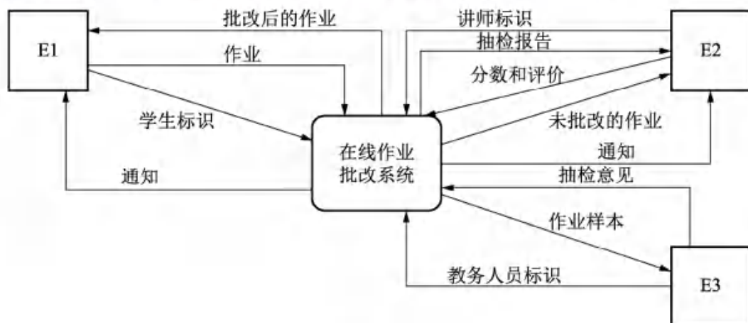
图 6-3 上下文数据流图
