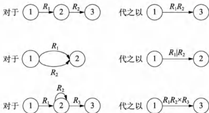
图 2-1 状态转换图(消去中间节点)
