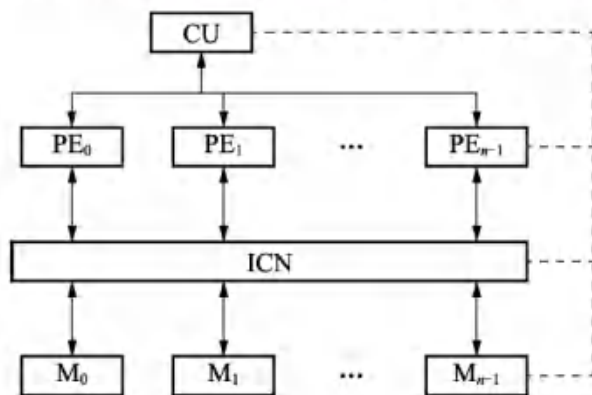
图 1-4 具有共享存储器的 SIMD 结构
