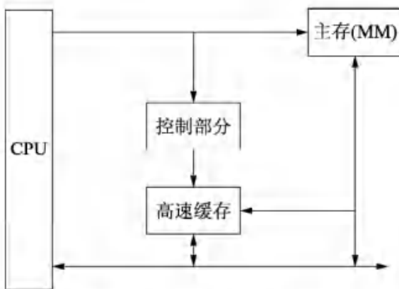
图 1-7 高速缓存的组成框图
