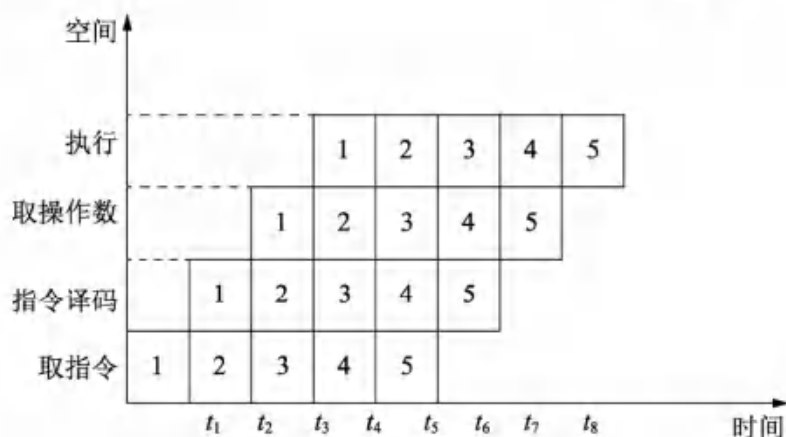
图 1-3 流水处理的时空图
