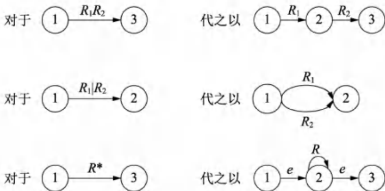
图 2-3 状态转换图(加入新节点)
