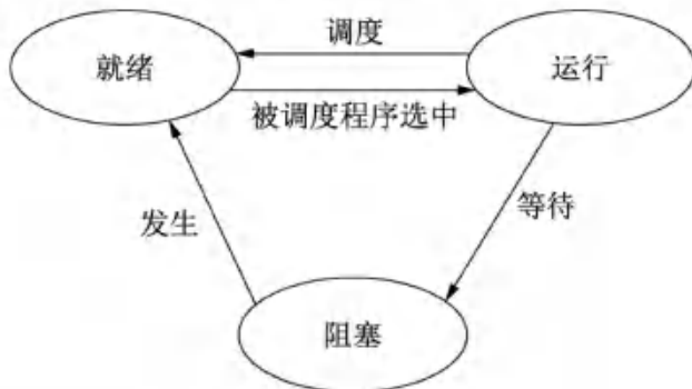
图4-1 进程的状态及其转换
