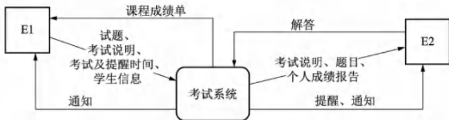
图 6-5 上下文数据流图
