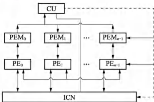
图 1-5 具有分布存储器的 SIMD 结构
