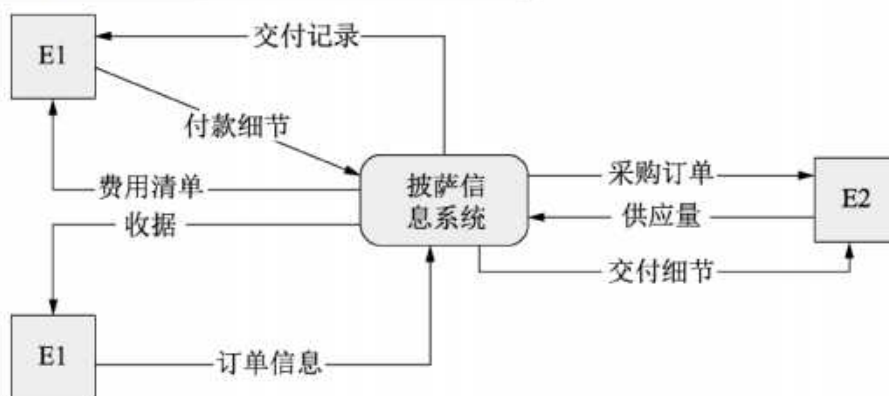
图 6-7 上下文数据流图
