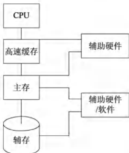
图 1-6 存储器层次结构示意图
