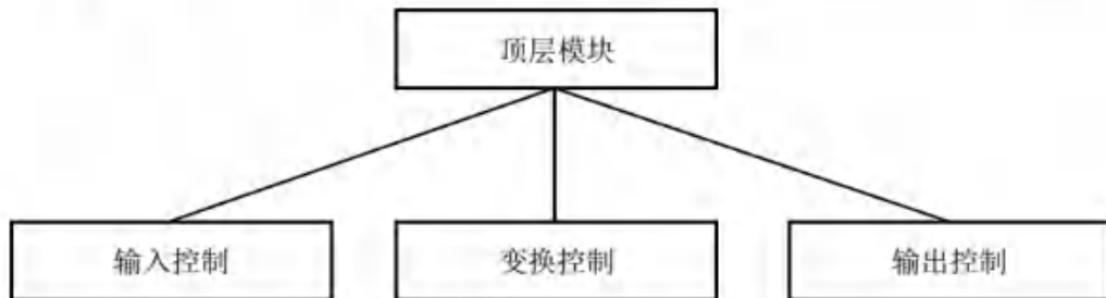
图 6-10 变换分析的第一级分解
