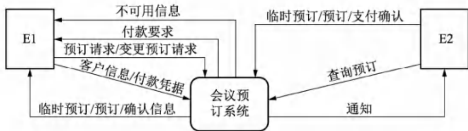
图 6-1 上下文数据流图
