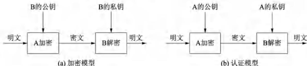
图 1-9 非对称加密的体制模型
